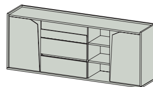
HA-3002T Aparador con cajones y abatible. Medidas \varnothing 180 \times 70 \times 40 cm.
